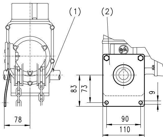
Fig. 1: Dispositivo ad inserimento momento torcente
