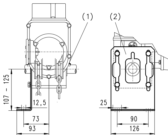
Fig. 2: Dispositivo ad inserimento consolle di flangia
