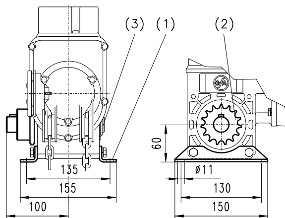
Fig. 3: Dispositivo a catena
